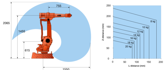
IRB 2400-10, IRB 2400-16
