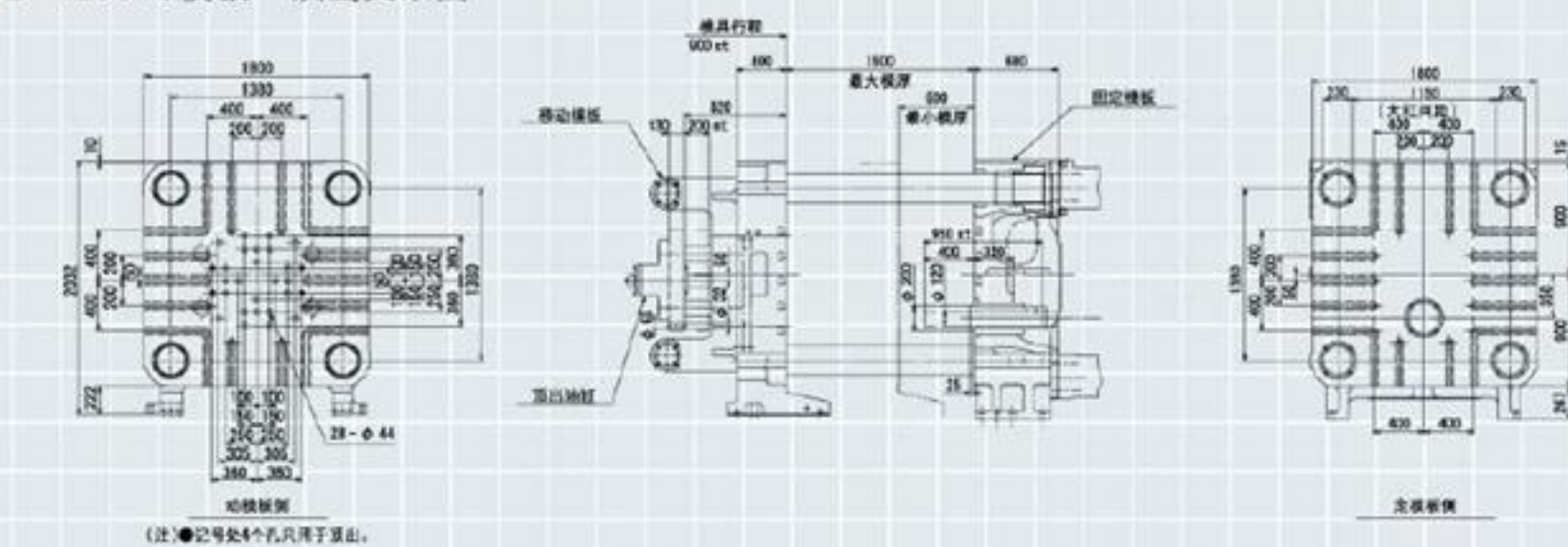
■BD-1250V5模板·顶出关系图
