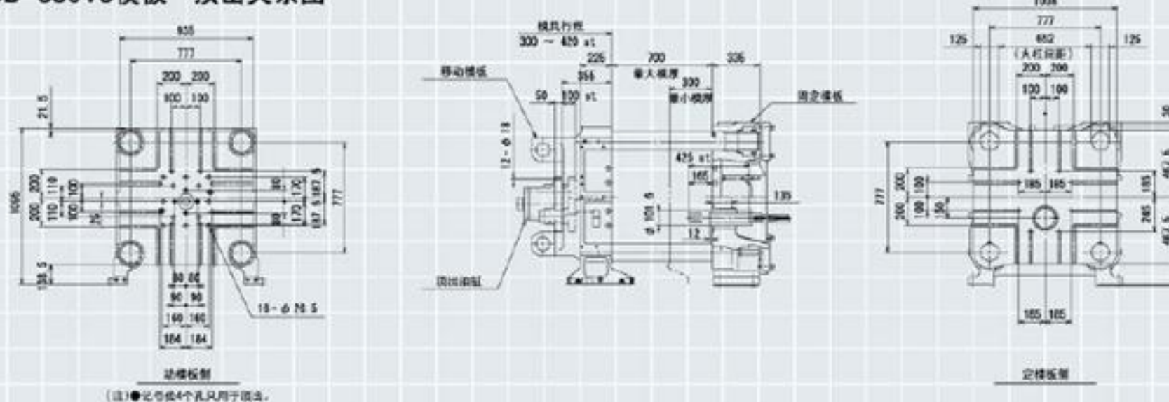
■BD-350V5模板·顶出关系图
