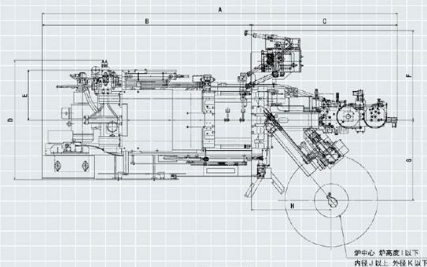
■BD-V5 系列外观图
