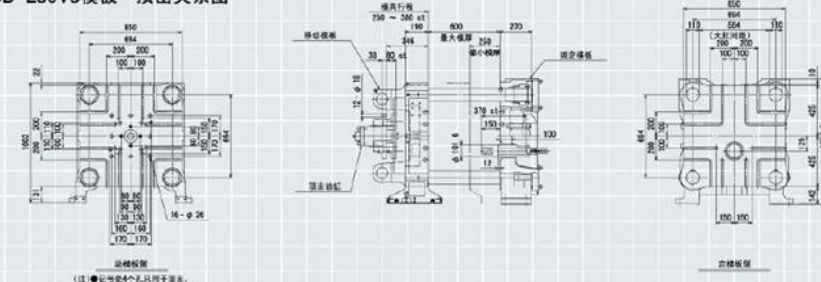
■BD-250V5模板·顶出关系图
