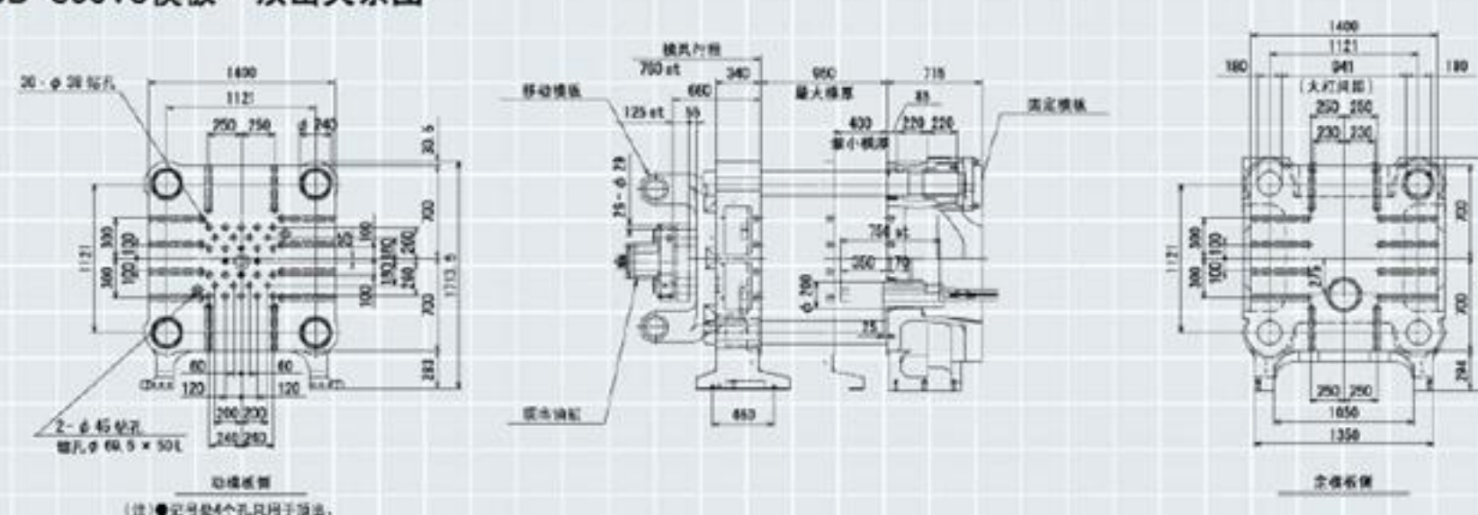
■BD-800V5模板·顶出关系图
