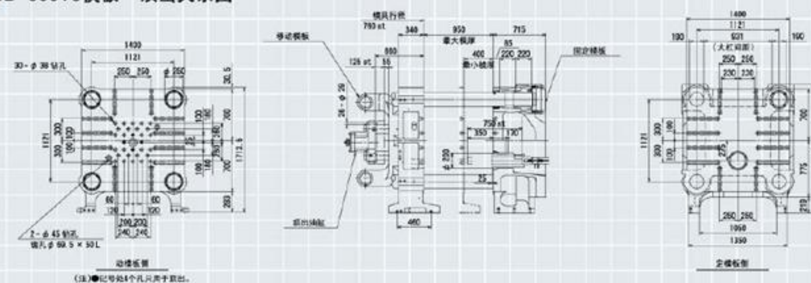
■BD-900V5模板·顶出关系图
