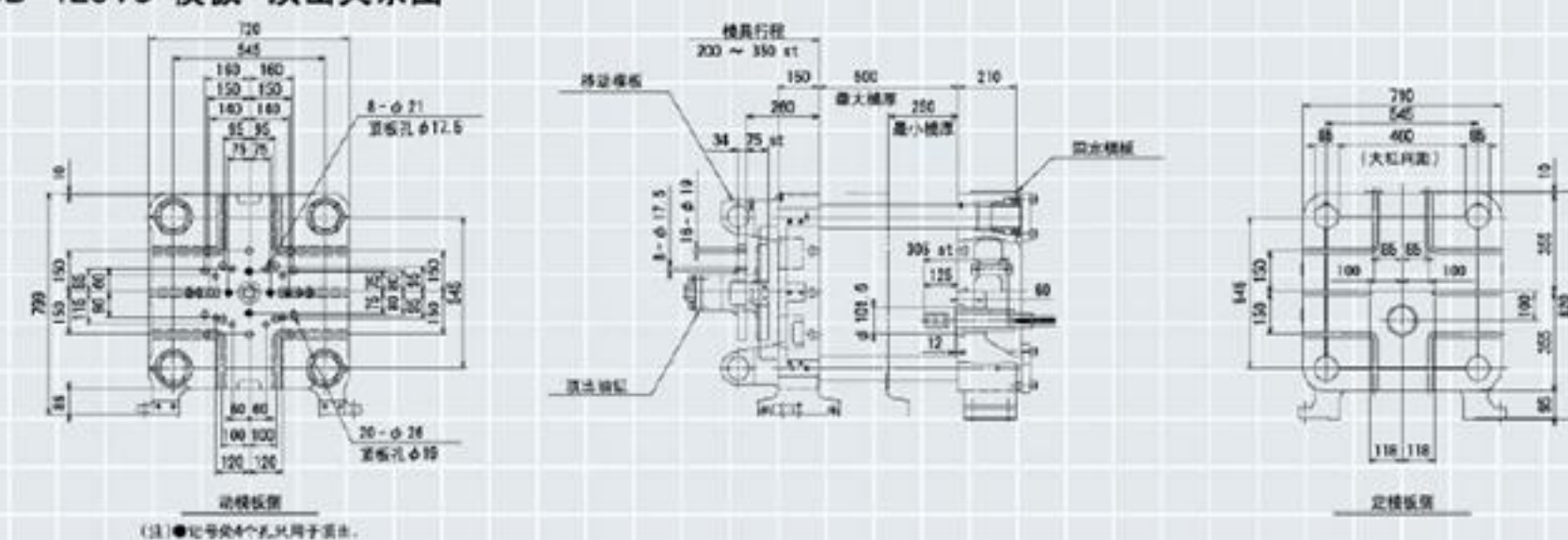
■BD-125V5 模板·顶出关系图
