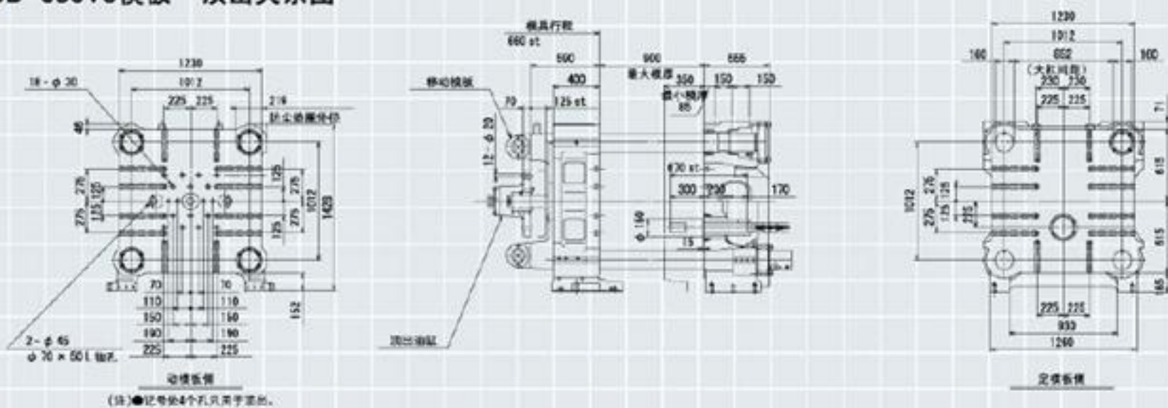
■BD-650V5模板·顶出关系图
